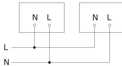
aansluitschema master/master
